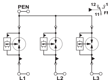
Электрическая схема
