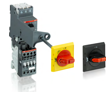
Монтажный комплект на дверь
