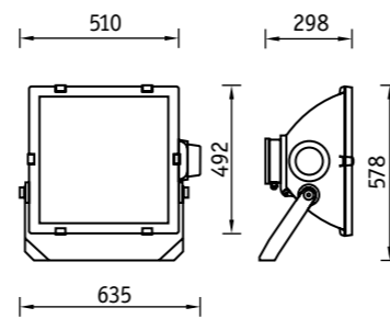
TERRA SM 2000H
