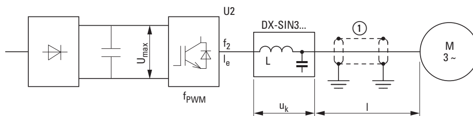
Рисунок 97: Наибольшая допустимая длина кабеля двигателя
