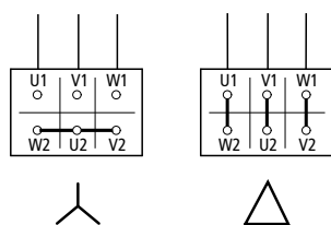
Рисунок 14: типы конфигурации: звезда слева, треугольник справа
