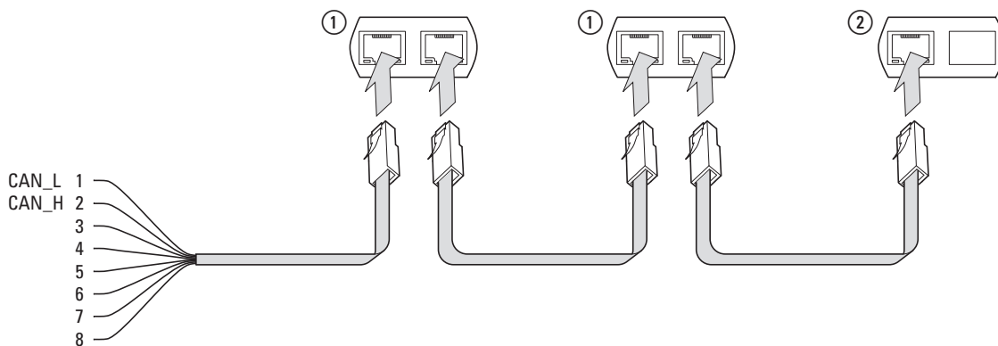
Рисунок 86: Оконечные резисторы шины
