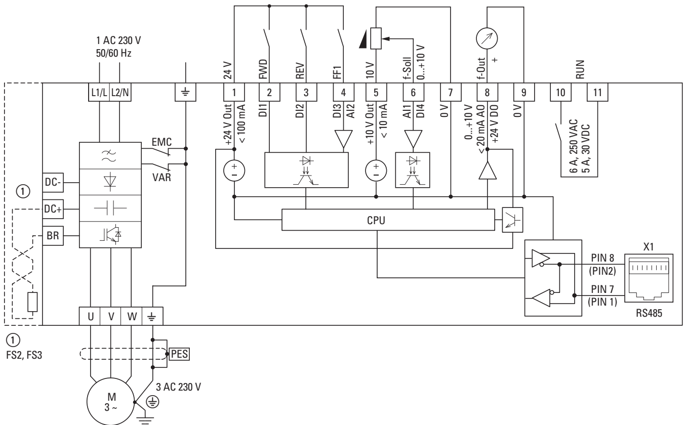
Рисунок 52: блок-схема DC1-12... Преобразователь частоты с однофазным напряжением сетевого питания и трехфазным напряжением двигателя
