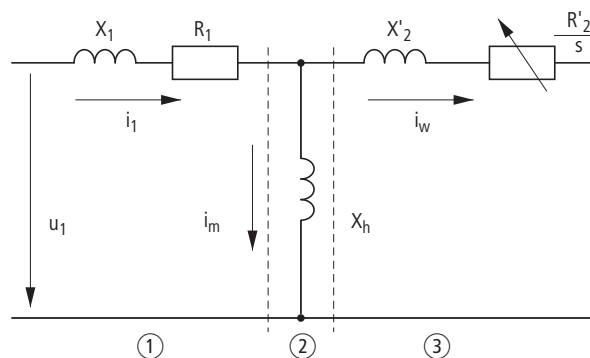
Рисунок 77: эквивалентная схема асинхронного двигателя.
