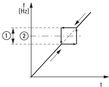
Рисунок 69: задание пропускаемой полосы частот ① P-26 ② P-27
