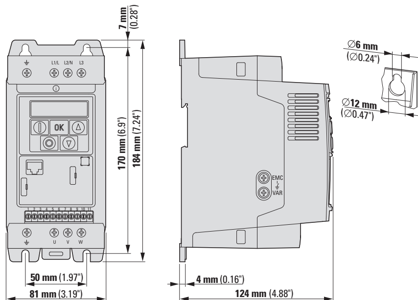
Рисунок 87: Типоразмер FS1
