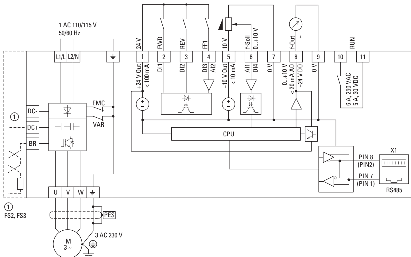
Рисунок 51: блок-схема DC1-1DxxxN...
