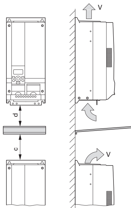
Рисунок 27: циркуляция воздуха с установленными воздушными заслонками
