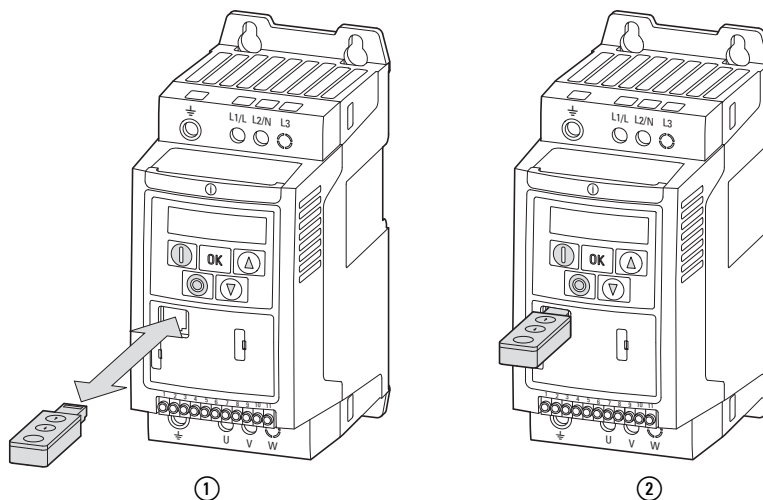
Рисунок 90: Установка DX-COM-STICK
