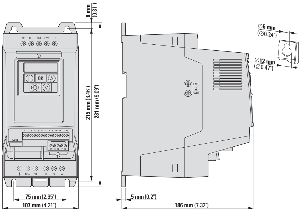
Рисунок 88: Типоразмер FS2
