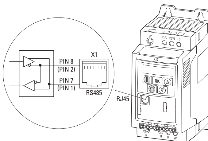
Рисунок 50: интерфейс RJ 45
