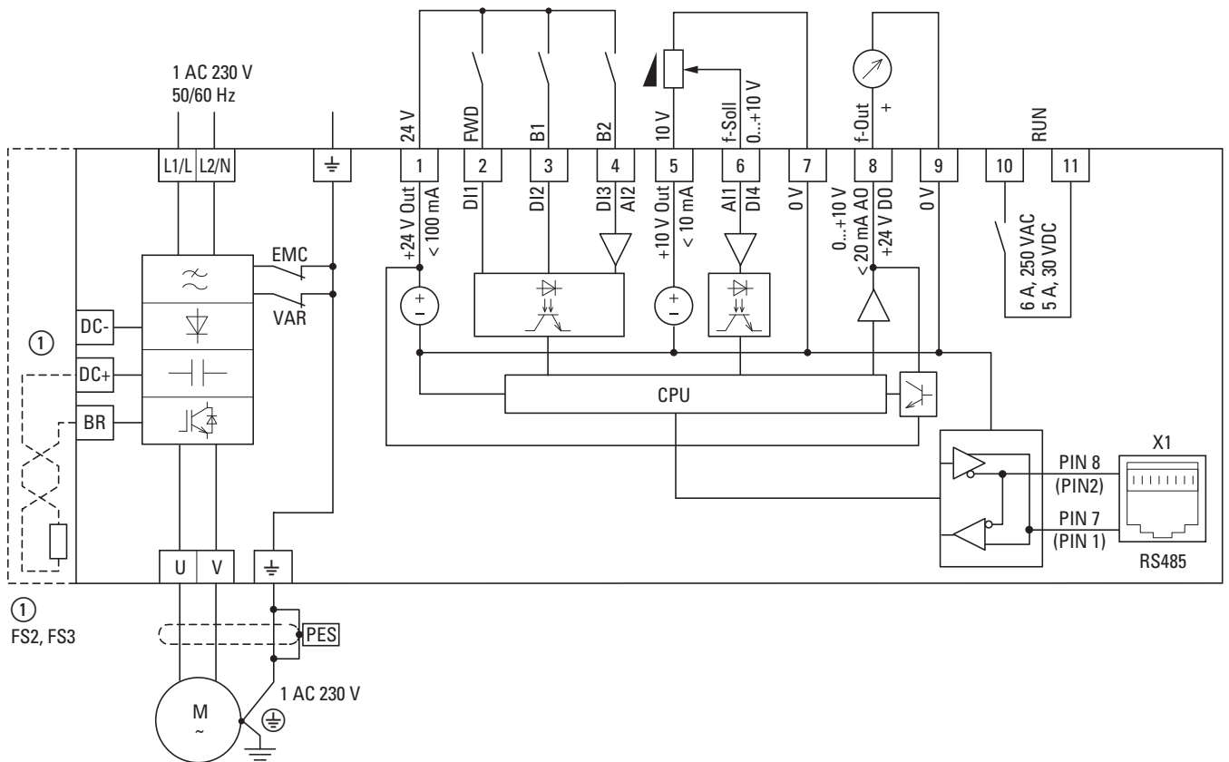
Рисунок 54: блок-схема DC1-S2...
