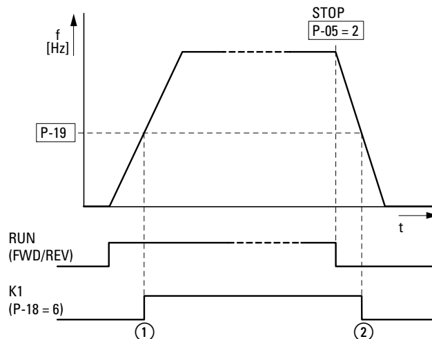
Рисунок 80: приведение в действие внешнего тормоза через K1
