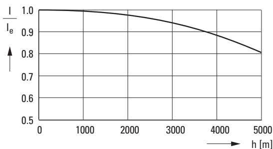
Рисунок 93: Изменение номинальных значений в зависимости от высоты эксплуатации установки над уровнем моря и температуры окружающей среды
