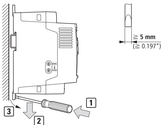
Рисунок 33: процедура снятия преобразователя с монтажной рейки
