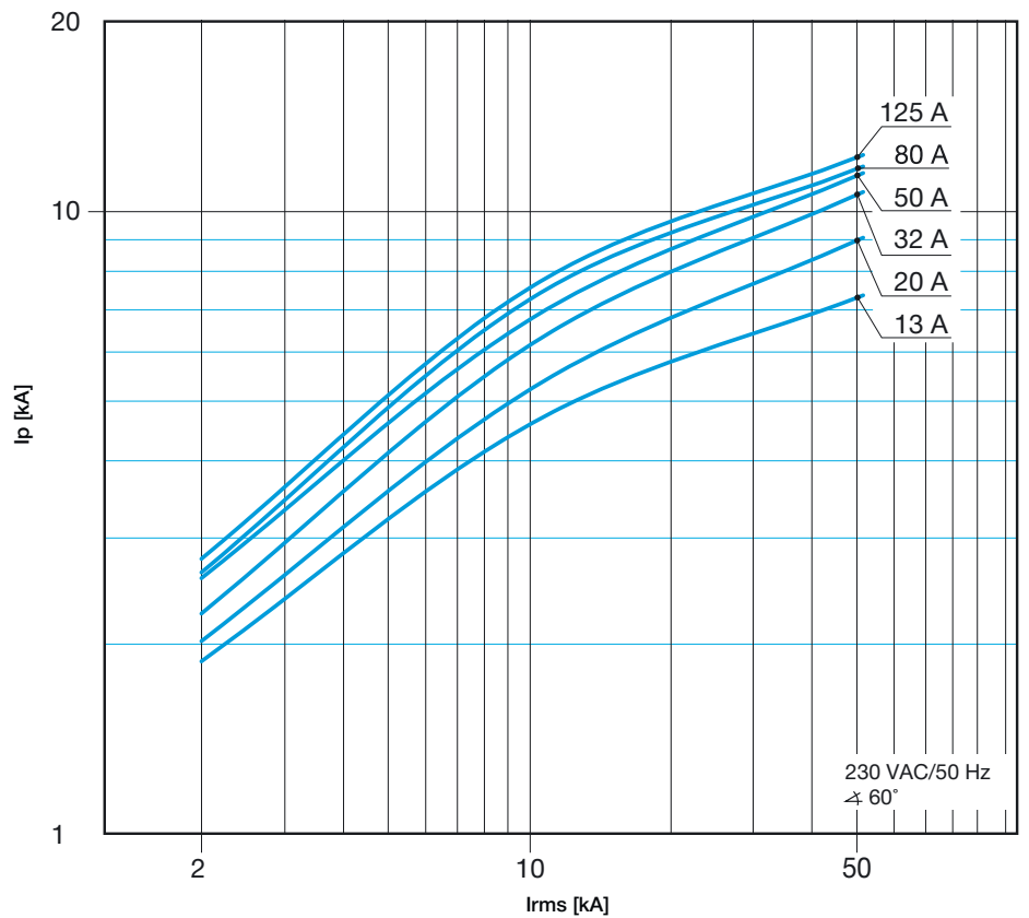
S 800 S характеристики B, C, D и K
