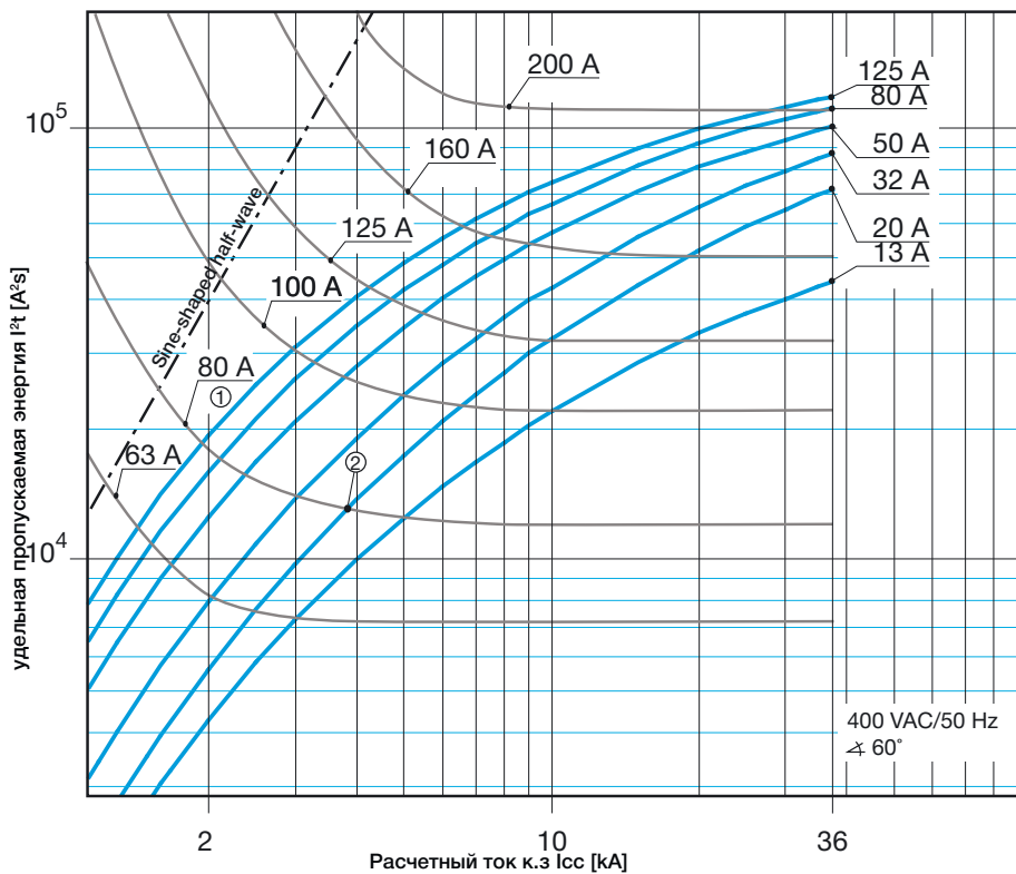
S800 N характеристики В, С и D 400 В удельная пропускаемая энергия
