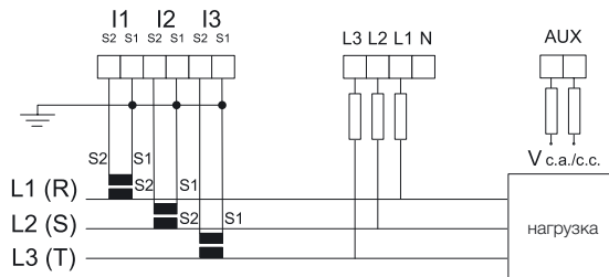
Трехфазная 3-проводная с 3-мя трансформаторами тока
