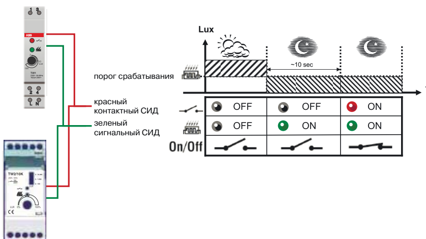
ТW1 и ТW2/10К принцип работы
