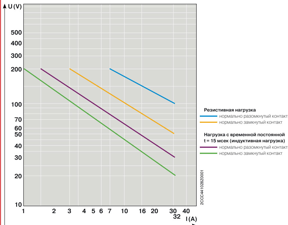
E 210 DC коммутационная способность
