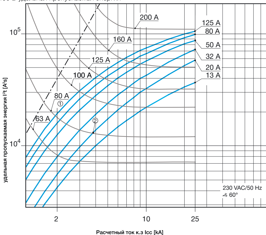
S800 C характеристики В, С, D и К 400 В удельная пропускаемая энергия
