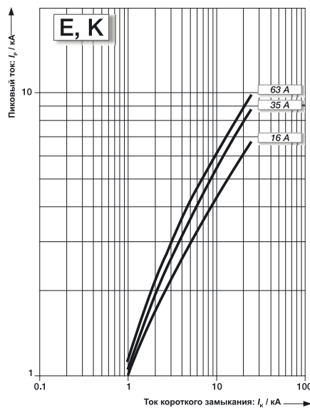
S750DR характеристики E и K ПИКОВЫЙ ТОК I_p
