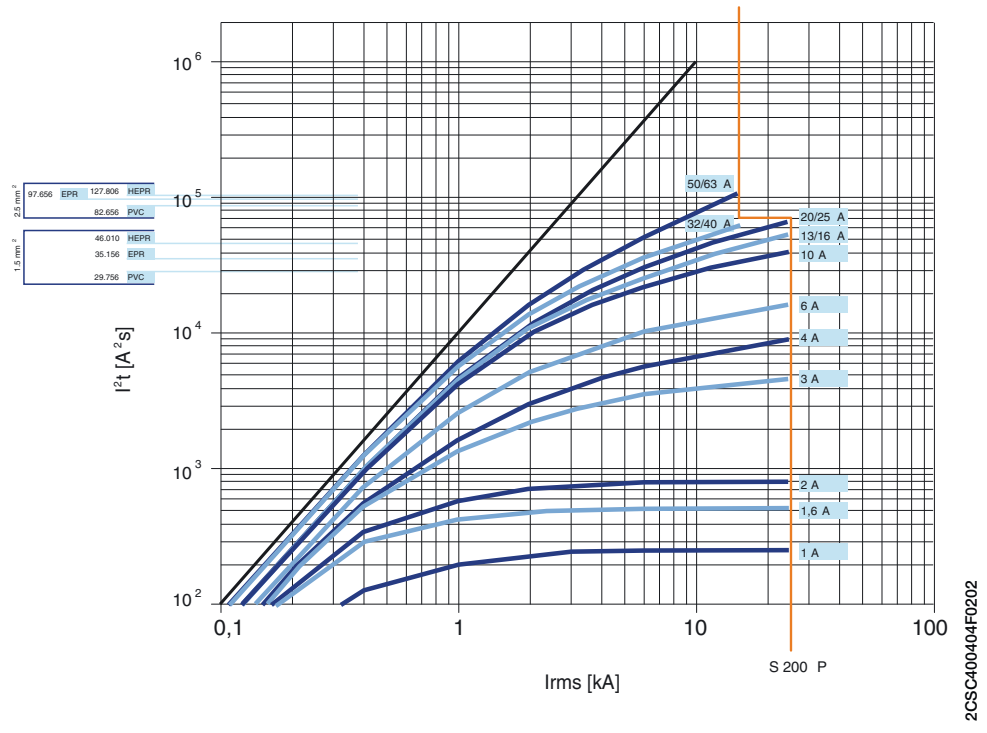
S 200 P, характеристика Z 230/400 В удельная пропускаемая энергия
