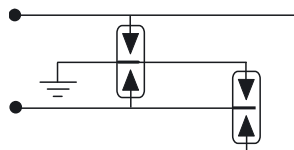
OVR TC 200 V при параллельном подключении
