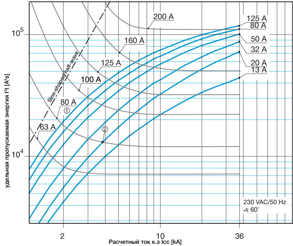
S800 N характеристики В, С и D 230 В удельная пропускаемая энергия
