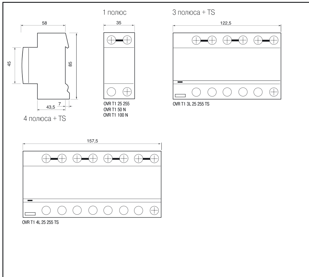
УЗИП Тип 1+2 ( I_{fi} = 15 \text{ кА} )
