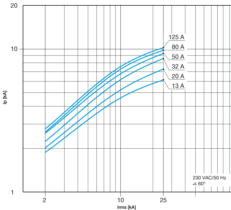
S 800 C характеристики B, C, D и K
