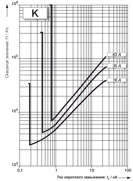
S750DR характеристика K удельная пропускаемая энергия
