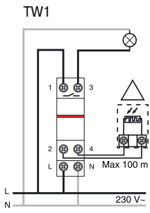
Схема подключения
