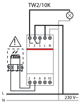
TW1 и TW2/10K принцип работы
