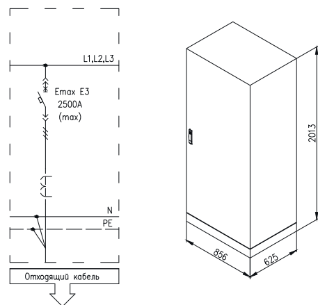
Распределительная панель DP-2500-2500-0001 / DP-2500-2500-0002
