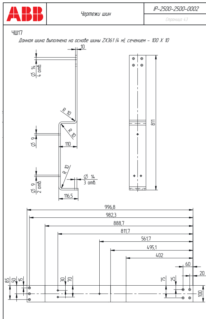
Рис. 1.2. Инструкция по обработке шины
