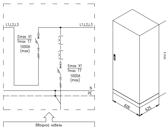
Распределительная панель DP-1000-M1000-0002 / DP-1000-M1000-0004
