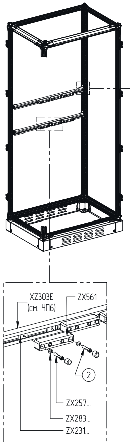
Рис. 1.11. Пример реализации опорных точек ошиновки аппарата
