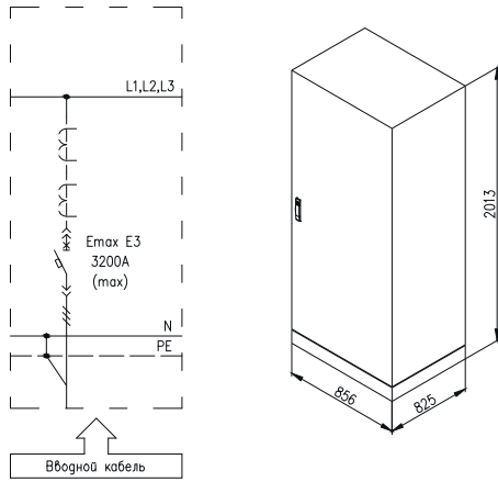
Вводная панель панель IP-3200-3200-1103
