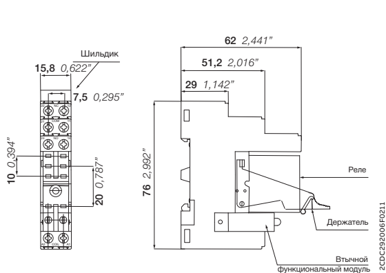
CR-PLS с винтовыми клеммами
