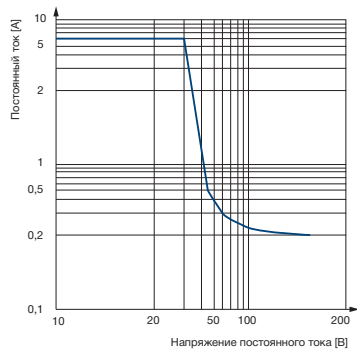
Макс. отключающая способность, нагрузка DC
