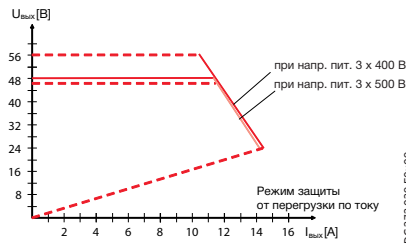
CP-T 48/10.0 Режим прерывания питания (hiccup mode) при перегрузке
