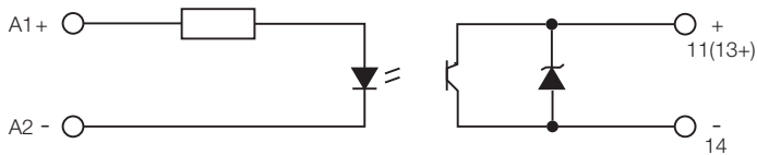
Оптопара CR-S с транзистором
