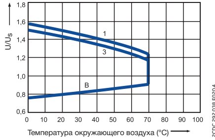
Диапазон рабочего напряжения и температуры катушки переменного тока
