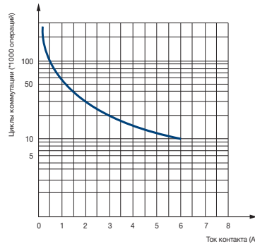
Кривая износоустойкости
