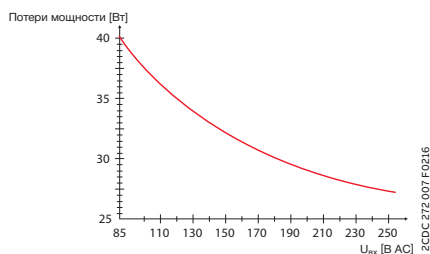
График зависимости средних потерь мощности (тепловыделения) от входного напряжения переменного тока
