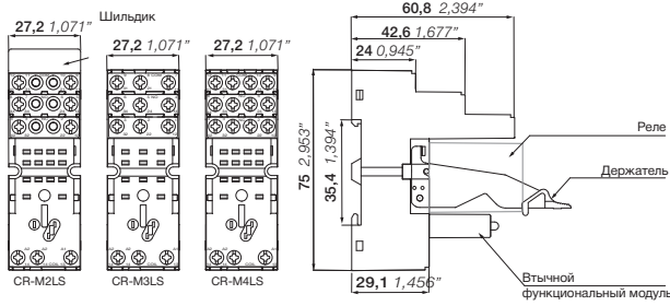
CR-M2LS — CR-M3LS — CR-M4LS с винтовыми клеммами
