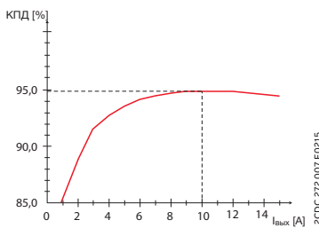
График зависимости среднего КПД от выходного тока
