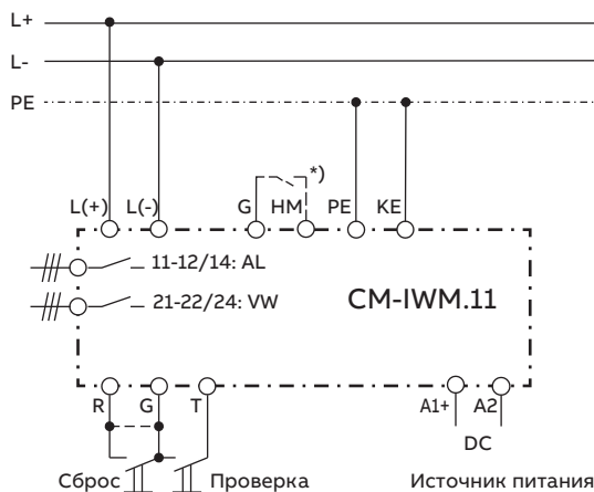
*) Подключение G-HM: измерительная цепь отключена
