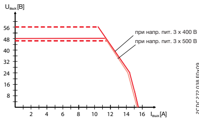
CP-T 48/10.0 Режим снижения напряжения при перегрузке
