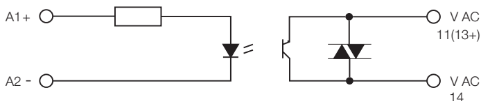
Оптопара CR-S с симистором
