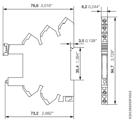
Цоколь CR-S с пружинными клеммами
