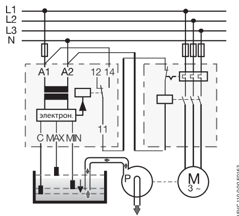
Контроль уровня жидкости — слив: выбрана функция ↓ (DOWN)
