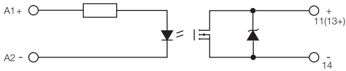
Оптопара CR-S с MOSFET-транзистором
