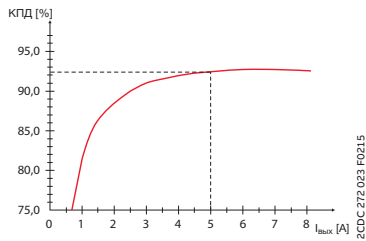
График зависимости среднего КПД от выходного тока
