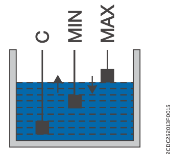
Режим работы с тремя электродами
