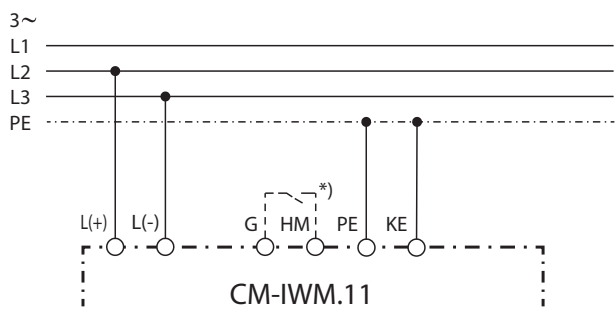
*) Подключение G-HM: измерительная цепь отключена
