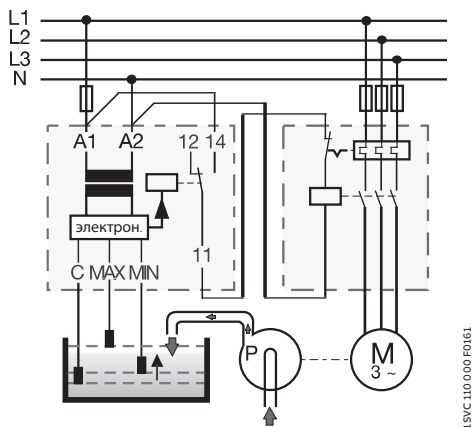
Контроль уровня жидкости — наполнение: выбрана функция ↑ (UP)
