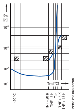
Характеристики термисторного датчика (РТС)
