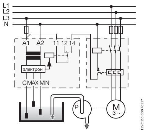
Контроль уровня жидкости — слив
