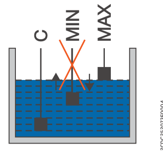
Режим работы с двумя электродами
