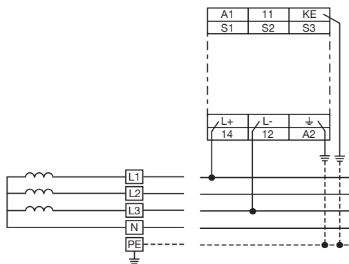
4-проводная сеть переменного тока
