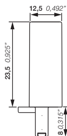
Функциональный модуль CR-P/Mxx
