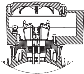
Соединительная коробка для двигателей типоразмеров 280 - 315
