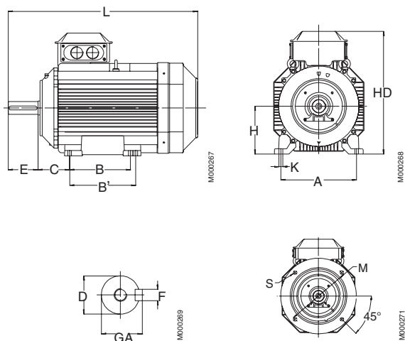
Типоразмеры 71-200
