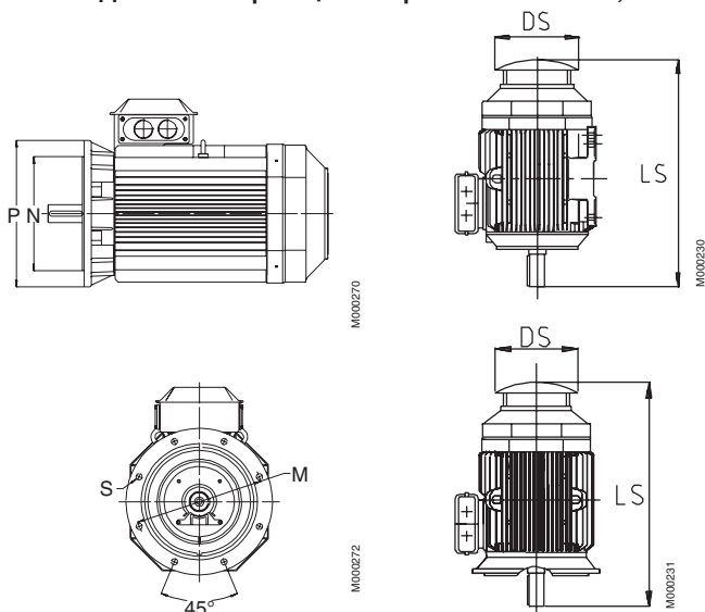
Защитный кожух, код модификации 005
