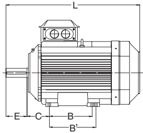
Двигатель с монтажом на лапах IM 1001, IM B3
