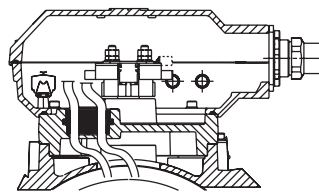
Соединительная коробка для двигателей типоразмеров 160 - 250
