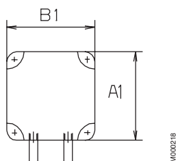
Двигатели типоразмеров 80 -132
