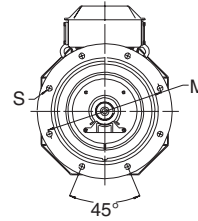
Типоразмеры 225-250
