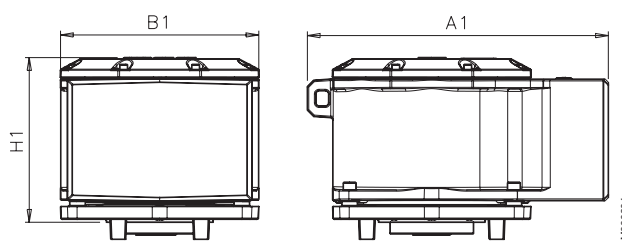
Двигатели EEx d, типоразмеры 355 - 400
