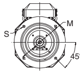
Типоразмеры 90-200
