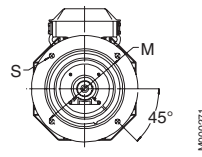
Фланцы
