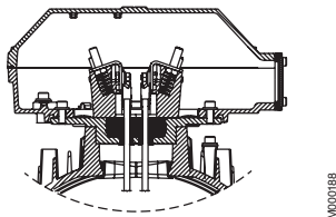
Соединительная коробка для двигателей типоразмеров 280 - 315
