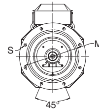
Типоразмеры 200-250
