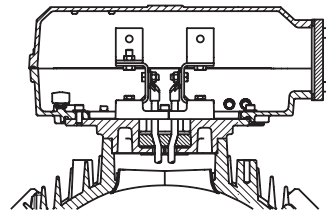
Соединительная коробка для двигателей типоразмеров 355 - 400
