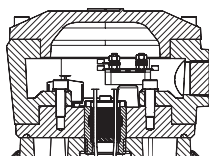
Соединительная коробка для двигателей типоразмеров 80 - 132
