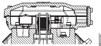
Соединительная коробка для двигателей типоразмеров 80 - 132
