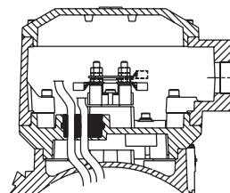
Соединительная коробка для двигателей типоразмеров 200 - 250
