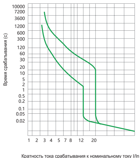
Кривая срабатывания
