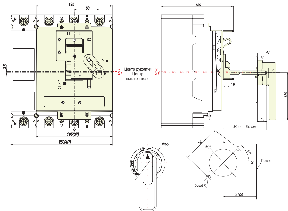
Габаритные и установочные размеры поворотной рукоятки SRH25-M8
