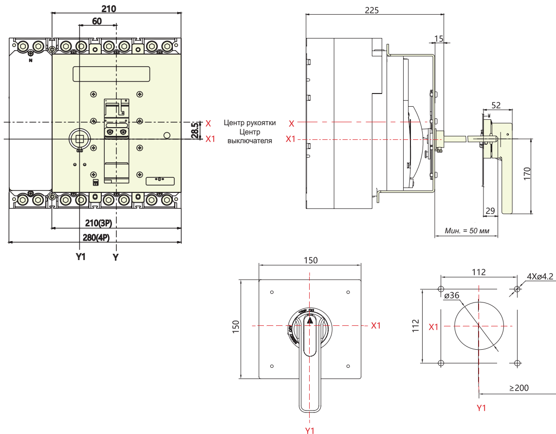
Габаритные и установочные размеры поворотной рукоятки SRH25-M8
