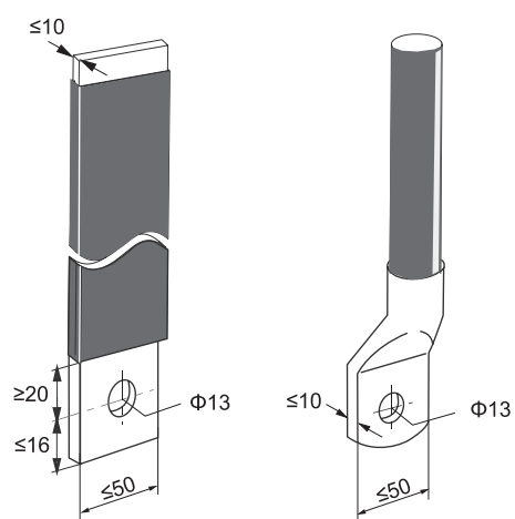
NM8N-800
