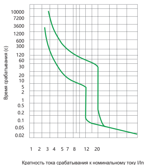
Кривая срабатывания
