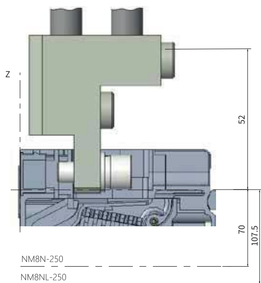
MC22-M8, 2 отверстия
