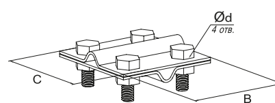
Зажим крестовидный (прут–прут)
