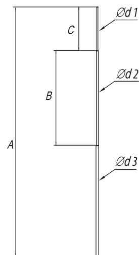
Мачты 8-10 метров
