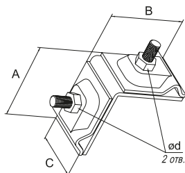
Держатель фальцевый
