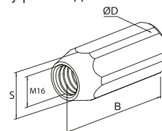
Муфта соединения
