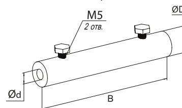
Зажим продольный
