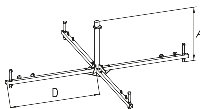
Четырёхнога
