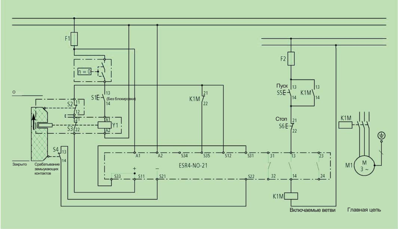
Устройство блокировки с защитным реле, 1 защитный позиционный выключатель, 2 размыкающих контакта/1 позиционный выключатель, 1 замыкающий контакт.
