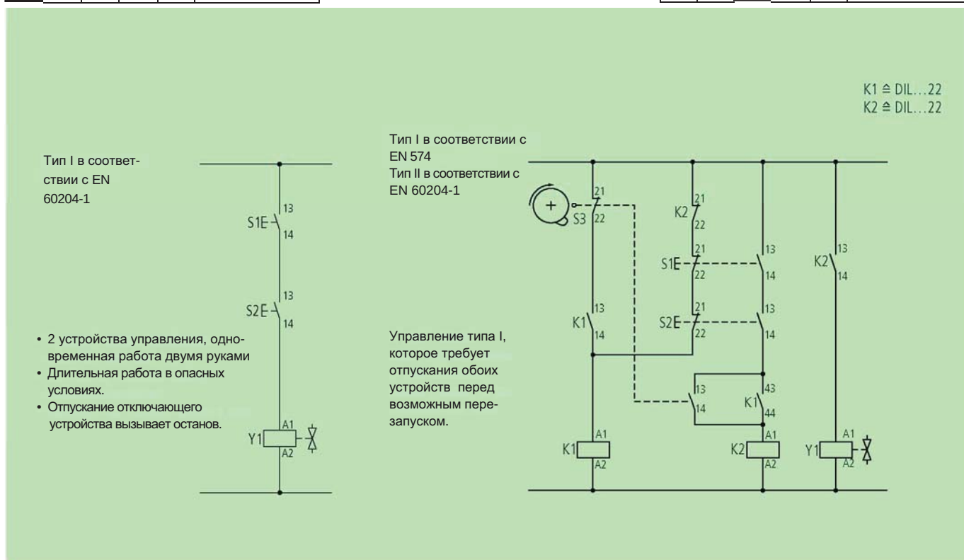
Двухручные органы управления типа I и II в соответствии с EN 60 204-1
