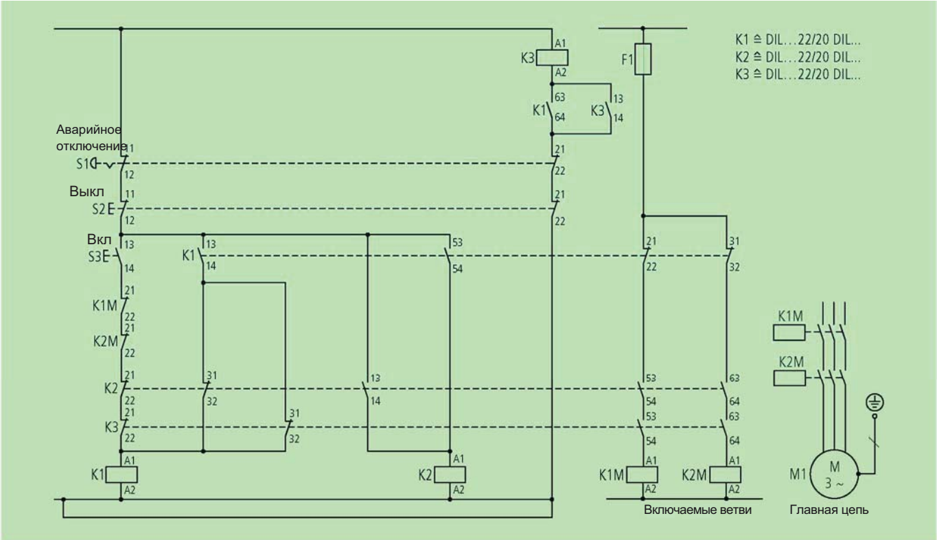
Аварийное отключение при контроле неисправностей кабеля питания
