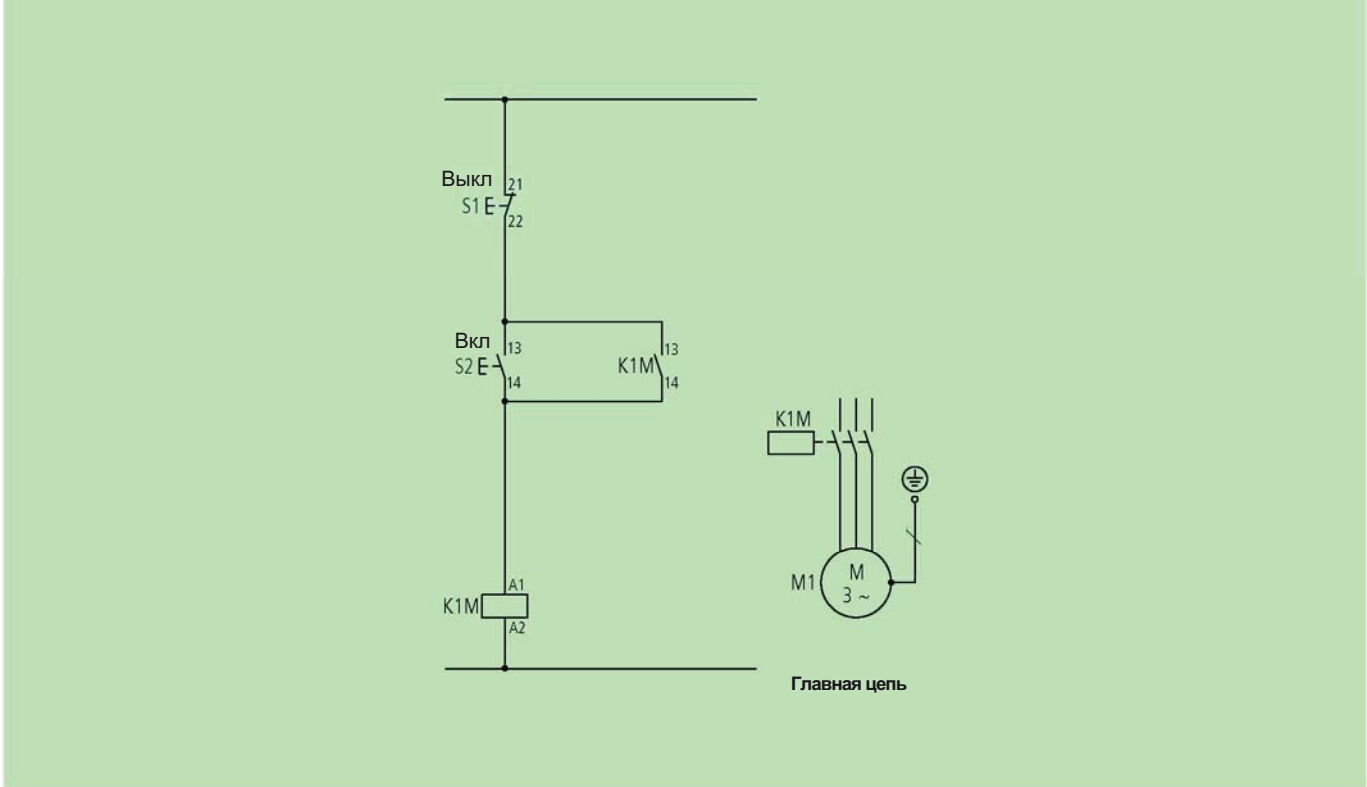
Самоудерживающийся контактор предотвращает перезапуск при восстановлении напряжения.
