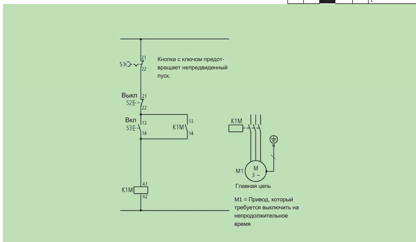
Предотвращение непредвиденного запуска с помощью кнопочного выключателя
