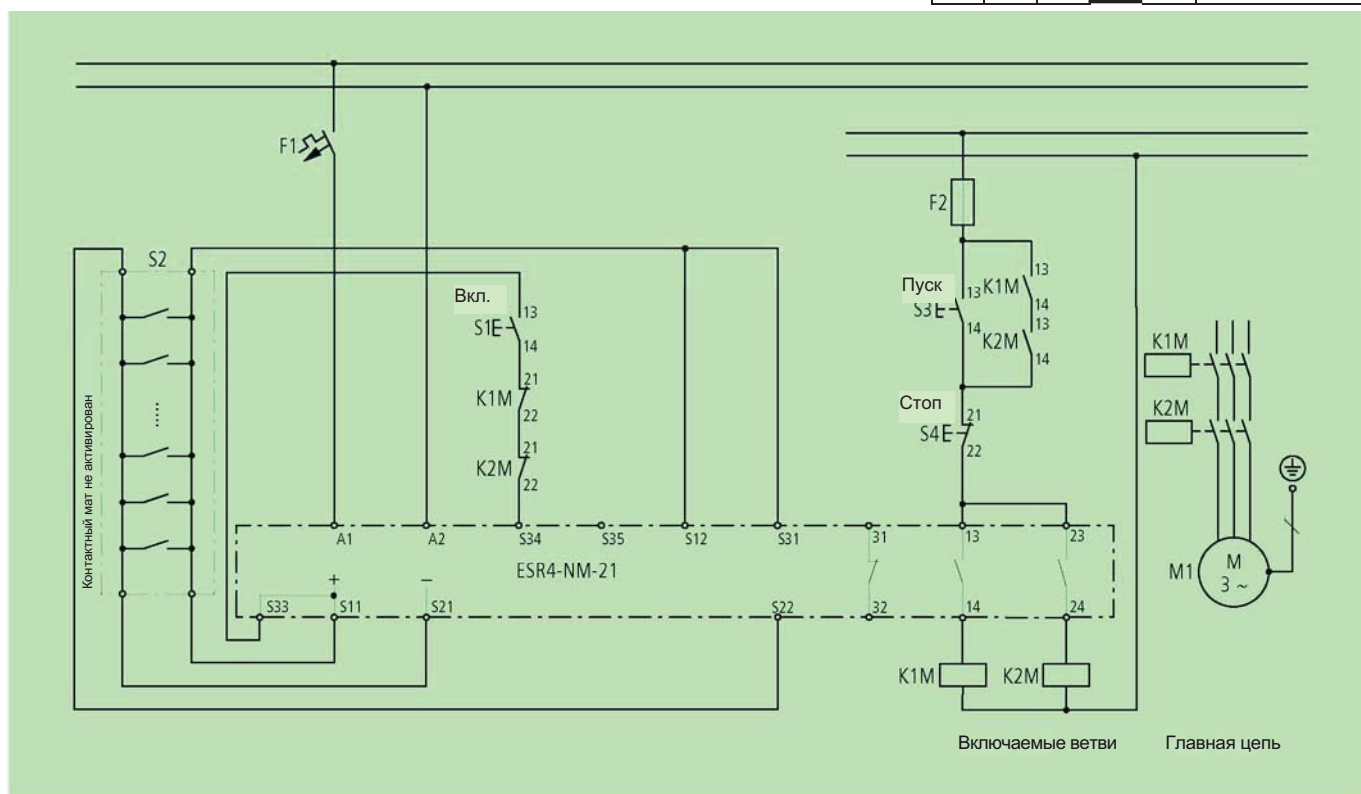
Контроль контактного мата, 4-полюсный контактный мат
