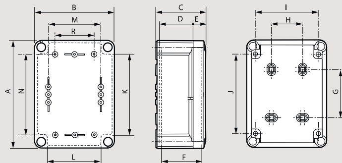
(1) Монтаж аксессуаров
