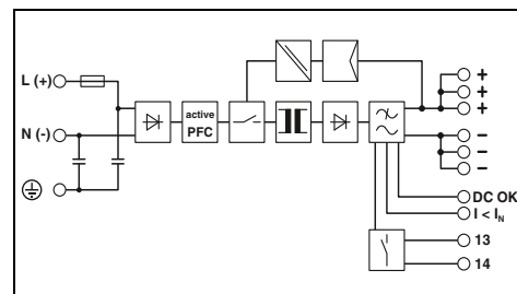
Источник питания, с лаковым покрытием, нанесенным окунанием, однофазный, 24 В пост. тока, 10 А
