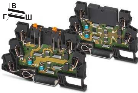
2 проводника, с общим опорным потенциалом
