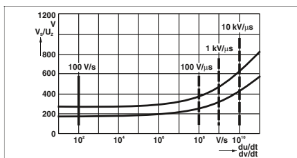
ВАХ газонаполненного разрядника
