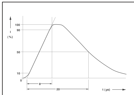
Импульс тока формы 8/20 согласно МЭК 60060-1
