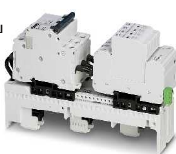
5-проводная система, L1, L2, L3, N, PE
