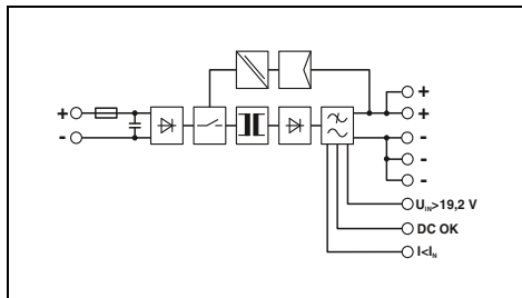
Преобразователи постоянного тока, с лаковым покрытием, нанесенным окунанием, 24 В пост. тока / 24 В пост. тока, 5 А
