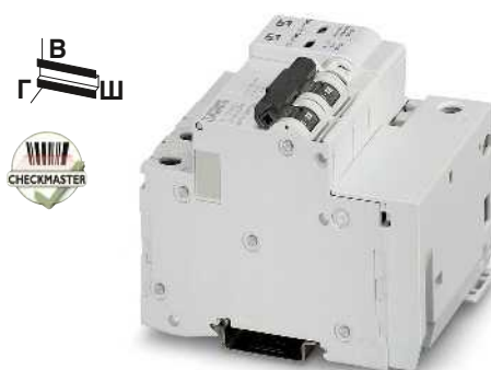
3-проводная система, L, N, PE
