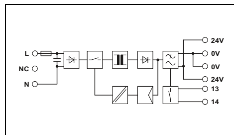
Источник питания, однофазный, 24 В пост. тока, 1,5 А, плоская конструкция, Опциональные соединители для установки на несущую рейку
