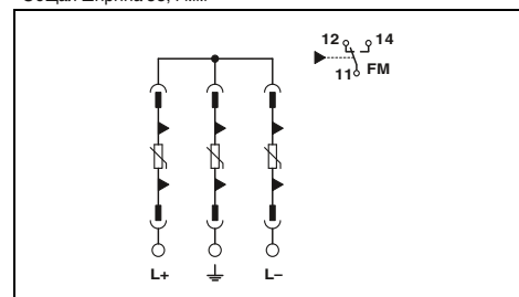
УЗИП класс для изолированных и заземленных с одной стороны фотогальванических систем
