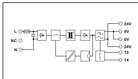
Источник питания однофазный, 24 В пост. тока, 1,5 А Опциональные соединители для установки на несущую рейку
