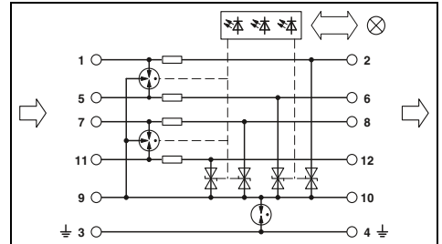
4 проводника, с общим опорным потенциалом, соединение 9/10 заземлено через газовый разрядник
