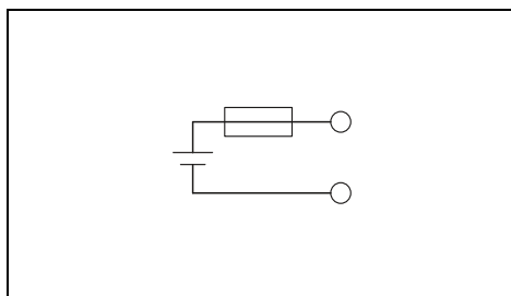
Энергоаккумуляторы, 12 В пост. тона, 1,6 Ач для MINI UPS 4 A
