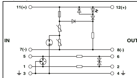
Комбинация защиты для пары сигнальных линий без потенциала земли и однофазной цепи питания
