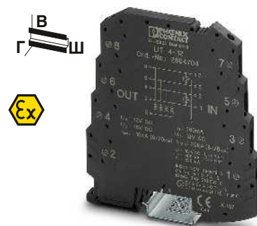
4 провода, без потенциала земли, без реактивных сопротивлений
