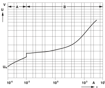
ВАХ металлооксидных варисторов
