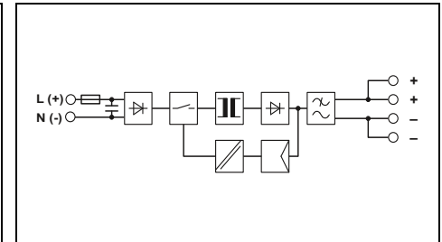
Источник питания, однофазный, 24 В пост. тока, 4,2 А
