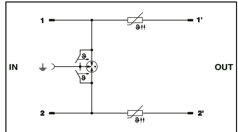
2 проводника, грубая защита, с отказоустойчивым контактом и токовой защитой (Powercross)
