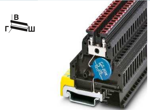
С варистором, направление действия: жила-земля
