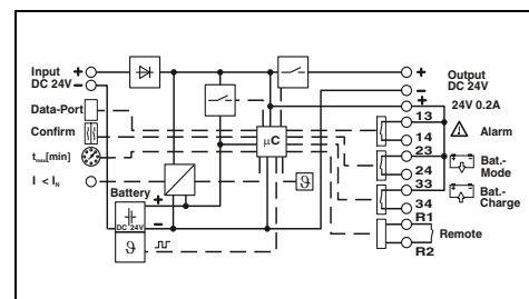
Источник бесперебойного питания со встроенным аккумулятором, 24 В пост. тока / 24 В пост. тока, 10 А, 3,4 Ач
