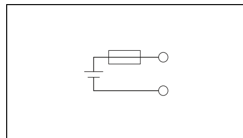
Энергоаккумуляторы, 24 В пост. тона, 0,8 Ач для MINI UPS 2 А
