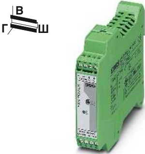
Источник питания, однофазный, 5 В пост. тока, 3 А
