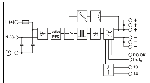
Источник питания, однофазный, 24 В пост. тока, 5 А
