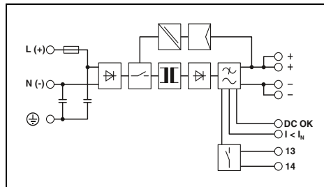
Источник питания, однофазный, 24 В пост. тока, 3,5 А
