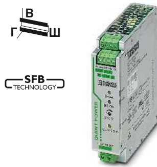
Преобразователь постоянного тока, 24 В пост. тока / 12 В пост. тока, 8 А
