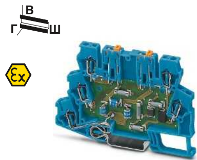
Витая пара (петля), искробезопасная цепь
