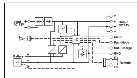
Источник бесперебойного питания со встроенным аккумулятором 12 В пост. тока / 12 В пост. тока, 4 А
