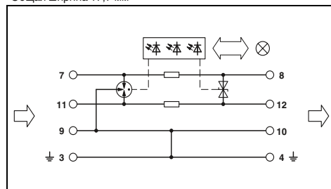
Витая пара (петля), без потенциала земли, соединение 9/10 заземлено напрямую
