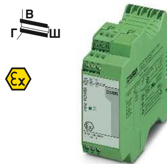
Источник питания однофазный, 24 В пост. тока, 1,5 А Опциональные соединители для установки на несущую рейку
