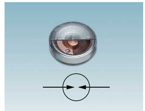
Герметичный разрядник с амплитудным ограничением
