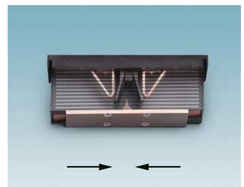
Искровые промежутки с дугогасящими пластинами
