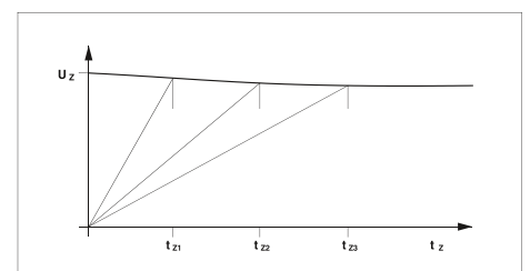
ВАХ искрового разрядника
