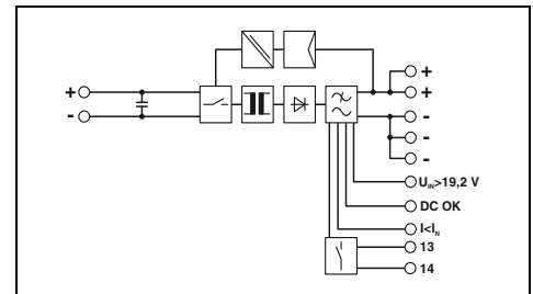
Преобразователи постоянного тока, с лаковым покрытием, нанесенным окунанием, 24 В пост. тока / 24 В пост. тока, 20 А
