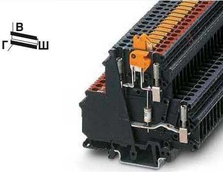
С супрессорным диодом, ножевым разделителем, направление действия: жила-жила
