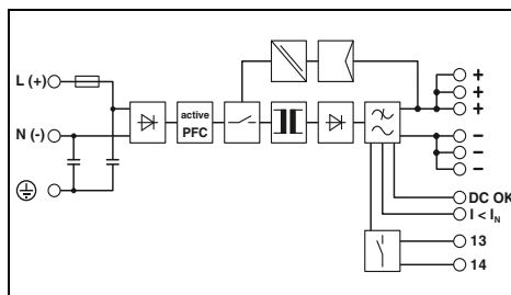
Источник питания, с лаковым покрытием, нанесенным окунанием, однофазный, 24 В пост. тока, 5 А
