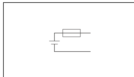
Энергоаккумуляторы, 12 В пост. тона, 2,6 Ач для MINI UPS 4 A
