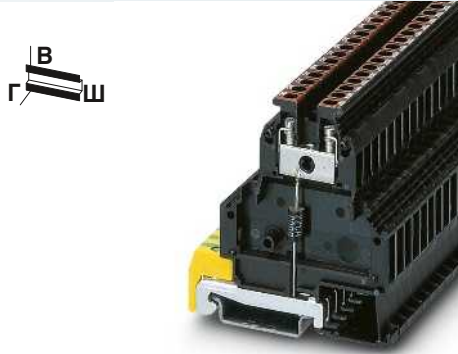
С супрессорным диодом, направление действия: жила-земля
