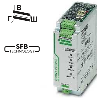
Преобразователь постоянного тока, 24 В пост. тока / 48 В пост. тока, 5 А
