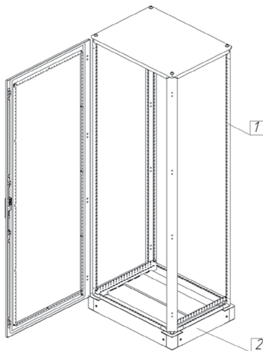
Распределительный шкаф
