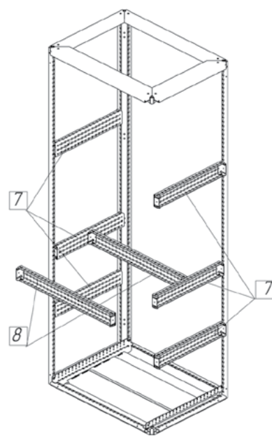
Система профилей
