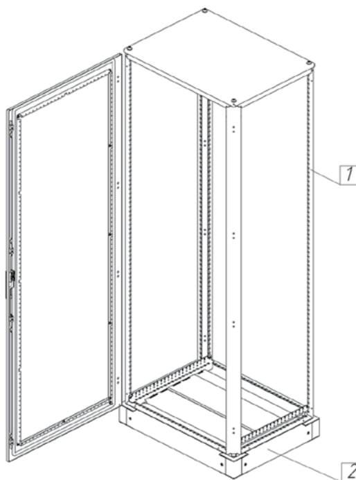
Система профилей
