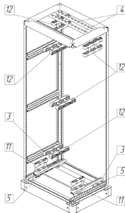
Шинные сборки
