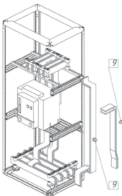
Шинные сборки
