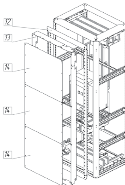
Пластронная система
