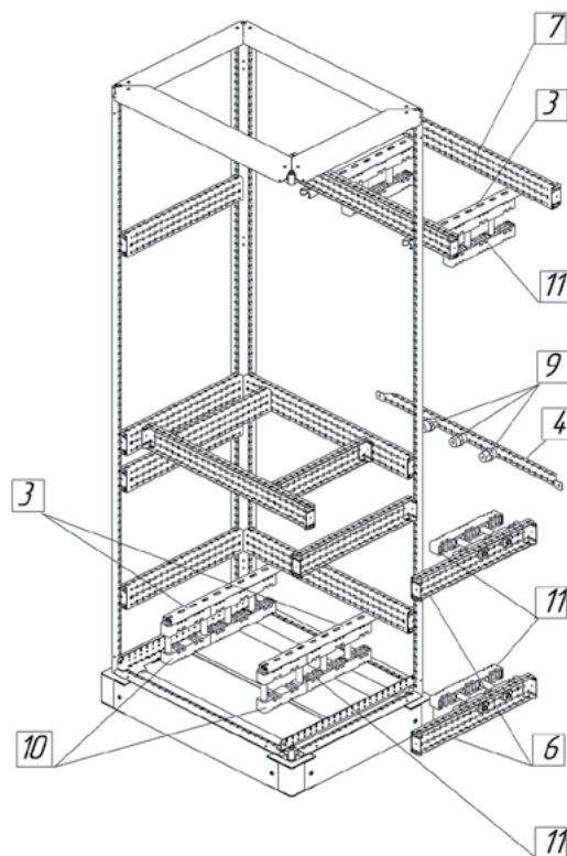
Шинодержатели
