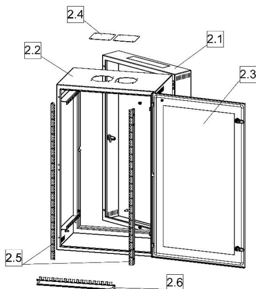
Шкаф трех-секционный
