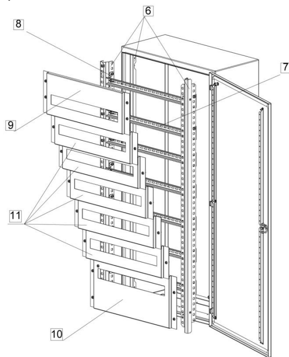
Наружные комплектующие
