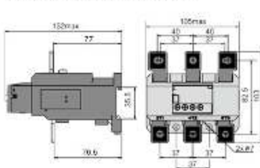
Независимая установка теплового реле MRG-105
