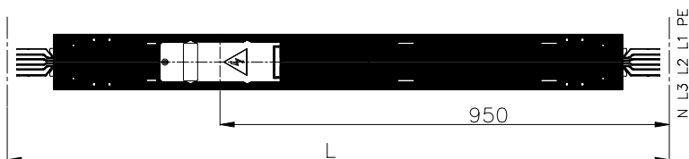
Транспортная секция с одной отводной розеткой 16-500А
