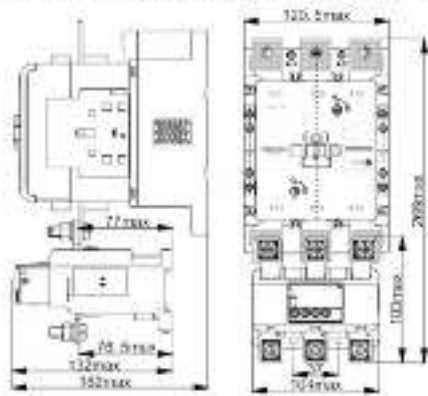
Комбинированная установка теплового реле MRG-105
