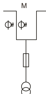
Ячейка измерения
